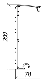
① Монтажный профиль
